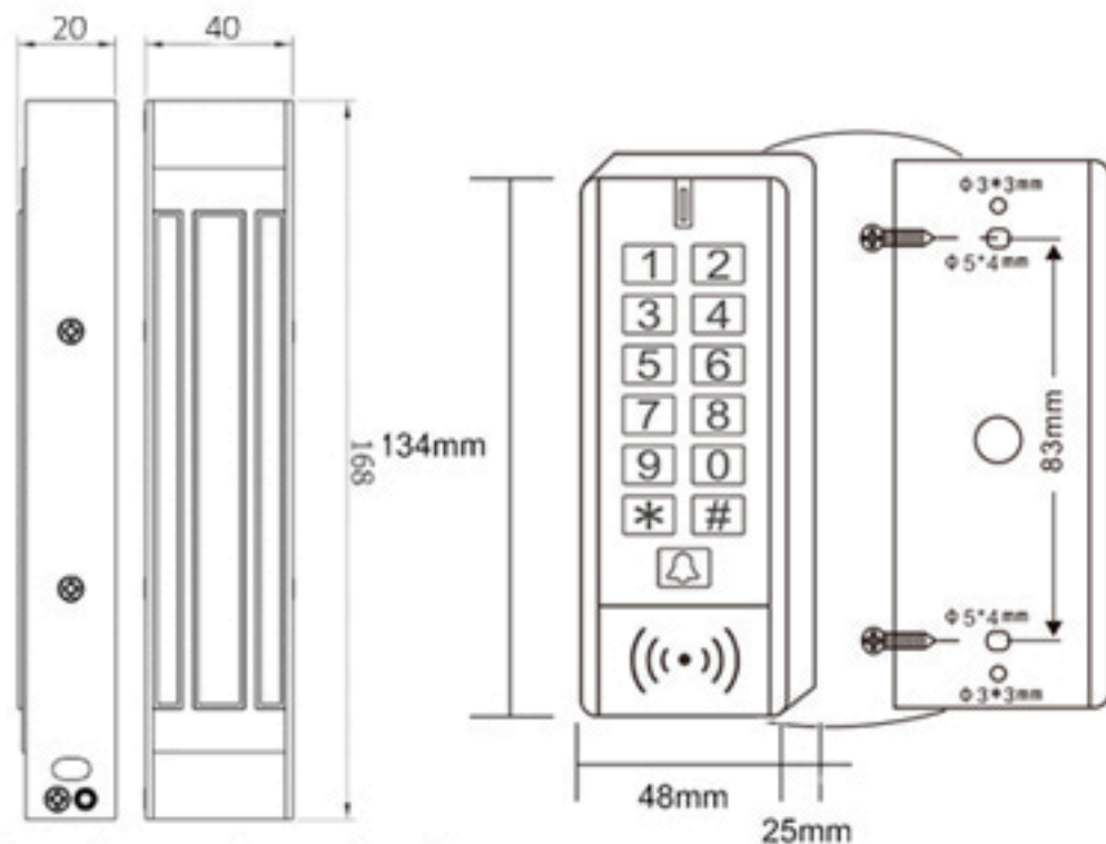
Fechadura Eletroímã
